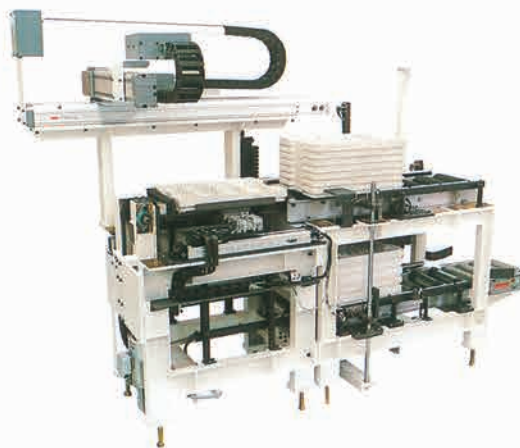
● 上段投入取出し下段払出しパレット パレット (490×350×H30) 7段積 ワーク取出し高さ1000m/m
