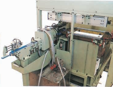
●多段標準型タイプ パレット(592×372×H49) 13段積 ワーク収納高さ1045m/m
