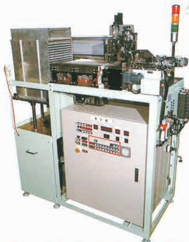
● マガジントレー特型 マガジントレー (430×330×H36) 26段積 ワーク充填高さ1370m/m
